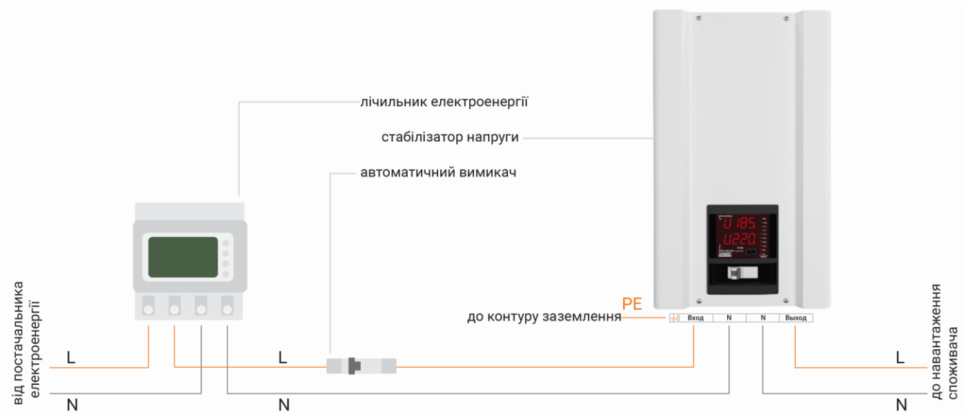
Рисунок 6. Схема підключення стабілізатора 25-80А до однофазної мережі
