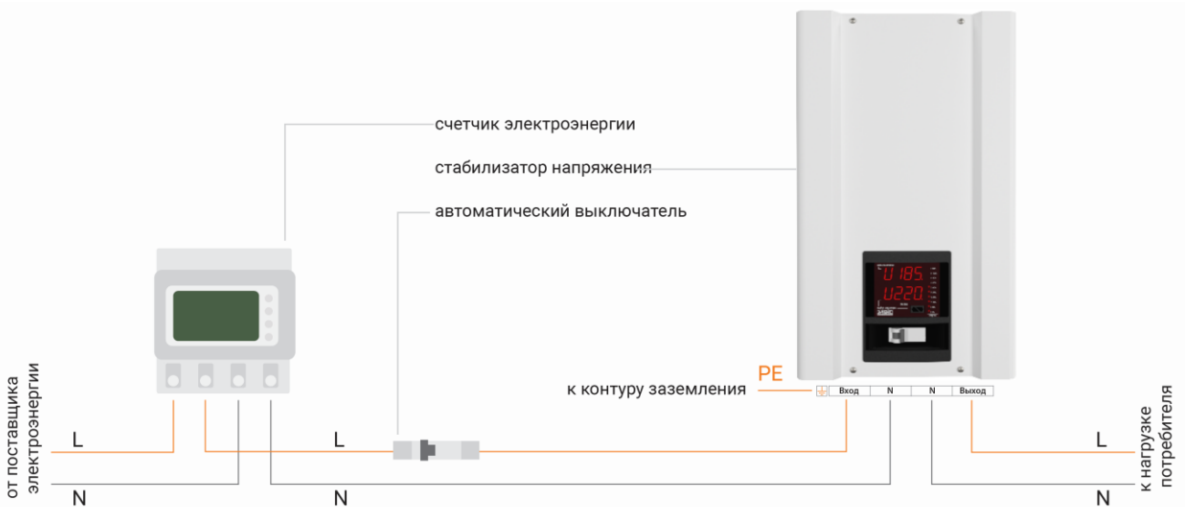
Рисунок 6. Схема подключения стабилизатора к однофазной сети
