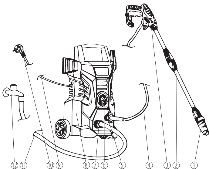
Рис. 1. Внешний вид 82-989
