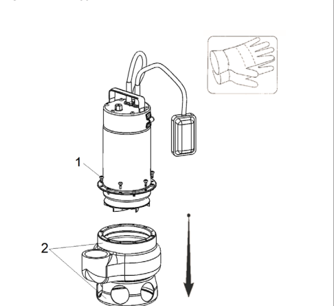
FIG. 4 • DAR DN50
