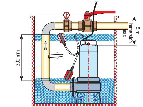
FIG. 4 • DAR DN50
