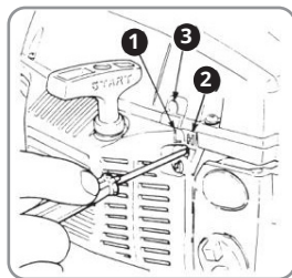
1.Голка L 2.Голка Н 3.Гвинт (Т) налаштування холостого ходу
