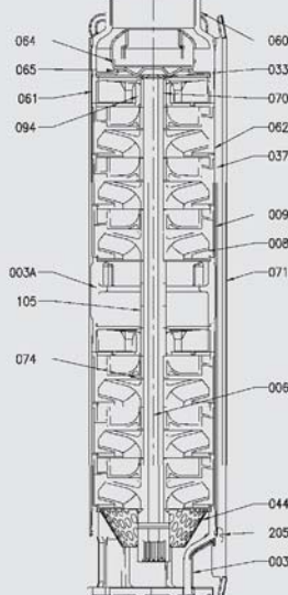
Помпа з подвійним кожухом
