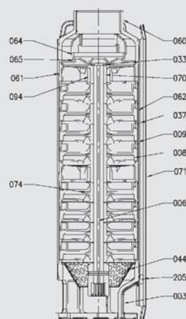
Помпа з одинарним кожухом
