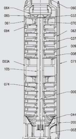
Помпа з подвійним кожухом
