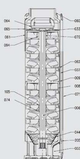
Помпа з одинарним кожухом
