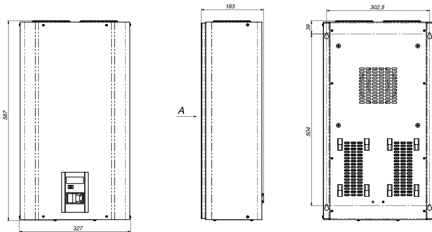
Рисунок 10. Габаритные и установочные размеры стабилизаторов АМПЕР-Р на 80А
