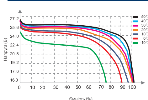
Крива розряду різної температури (0,2С)
